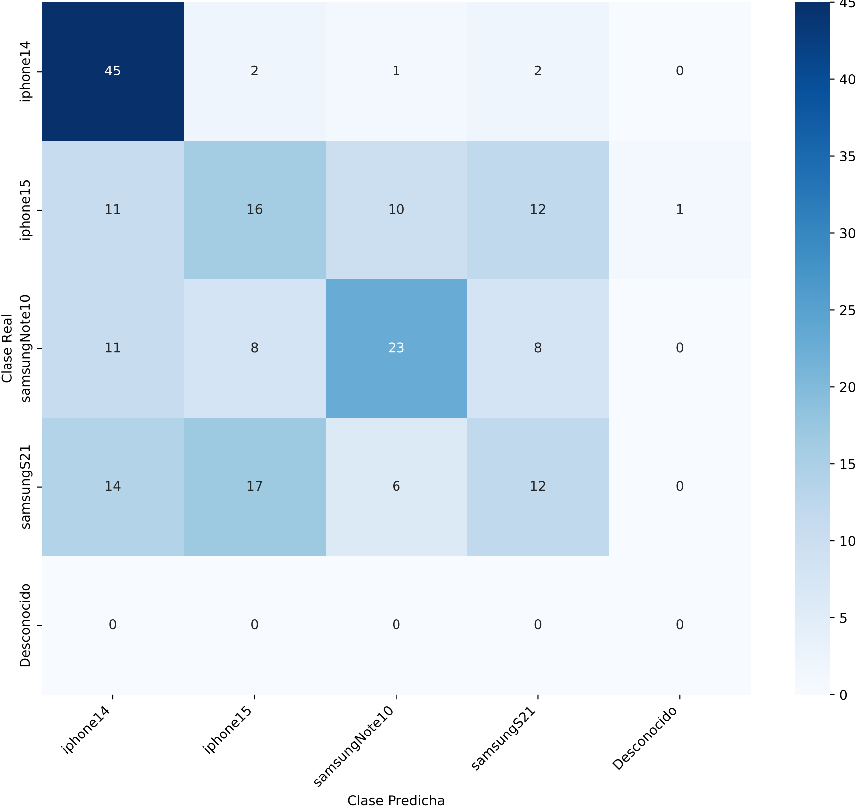
Matriz de Confusión - PRNU_FILTRO LINEAL
